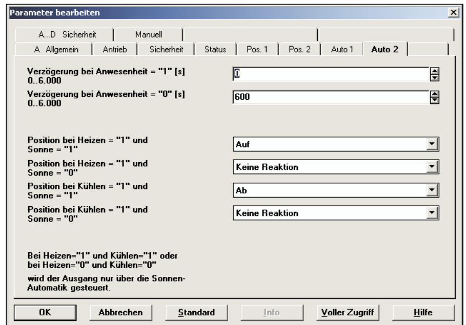
Abb. 35: Parameterfenster „Auto 2“
