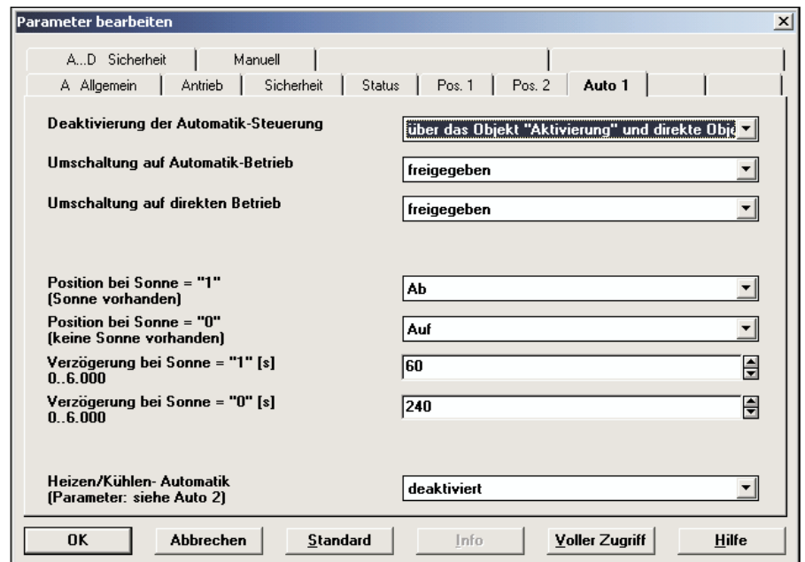
Abb. 34: Parameterfenster „Auto 1“
