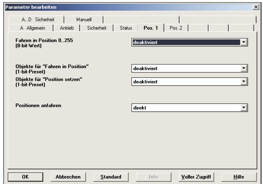
Abb. 32: Parameterfenster „Pos. 1“
