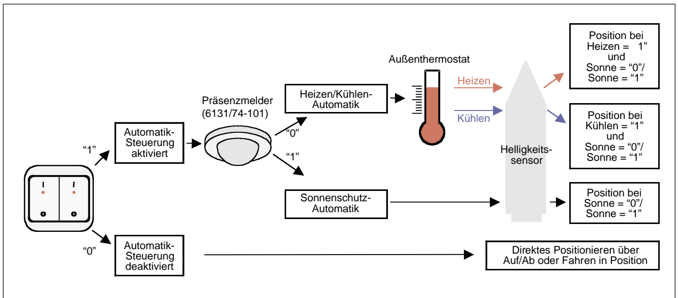
Abb. 13: Aufbau einer Heizen/Kühlen-Automatik-Steuerung
