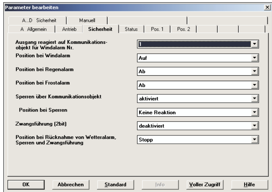
Abb. 30: Parameterfenster „Sicherheit“
