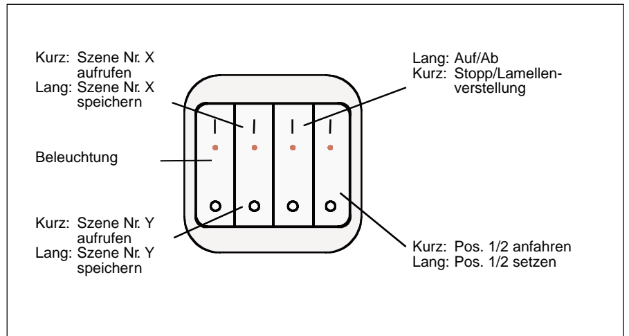
Abb. 16: Tasterbelegung Auf/Ab, Position anfahren, Position setzen
