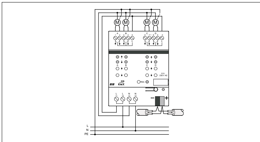
Abb. 15: Planung einer Spannungsüberwachung in den Schaltkreisen
