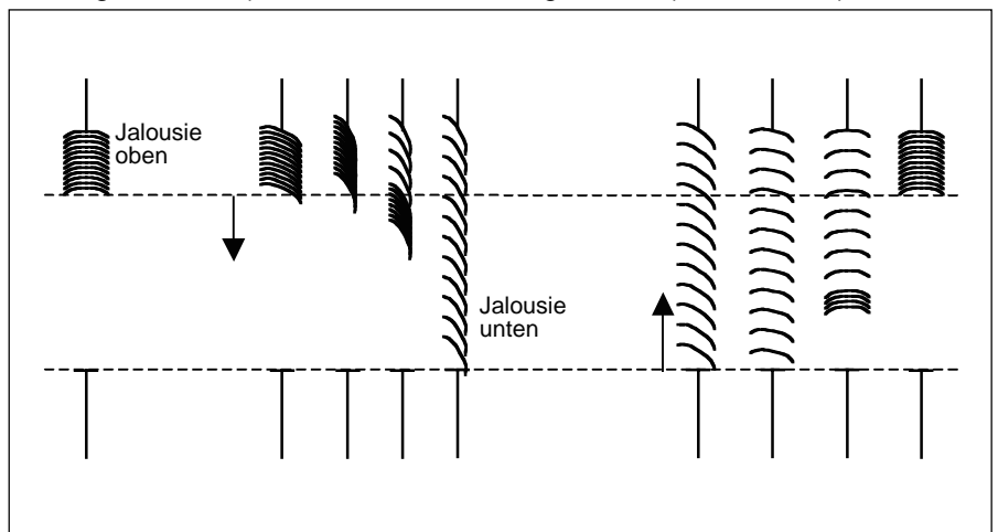
Abb. 2: Lamellenstellung beim Auf- und Abfahren der Jalousie
