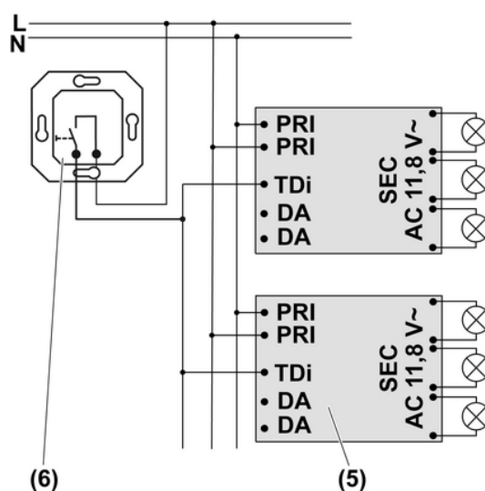
Imagen 5: Plano de conexiones con pulsador de instalación
